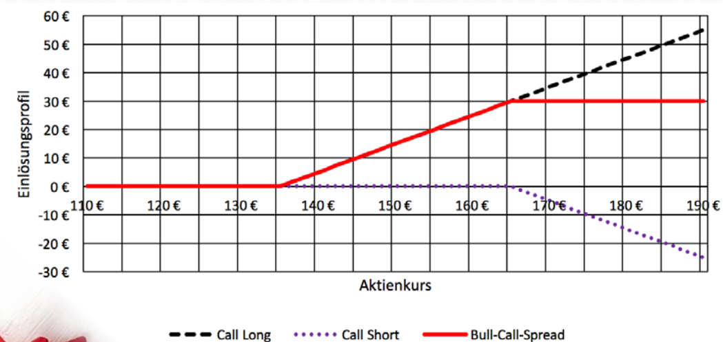
Darstellung 1: Einlösungsprofil Bull-Call-Spread zur Fälligkeit mit Call-Optionen
